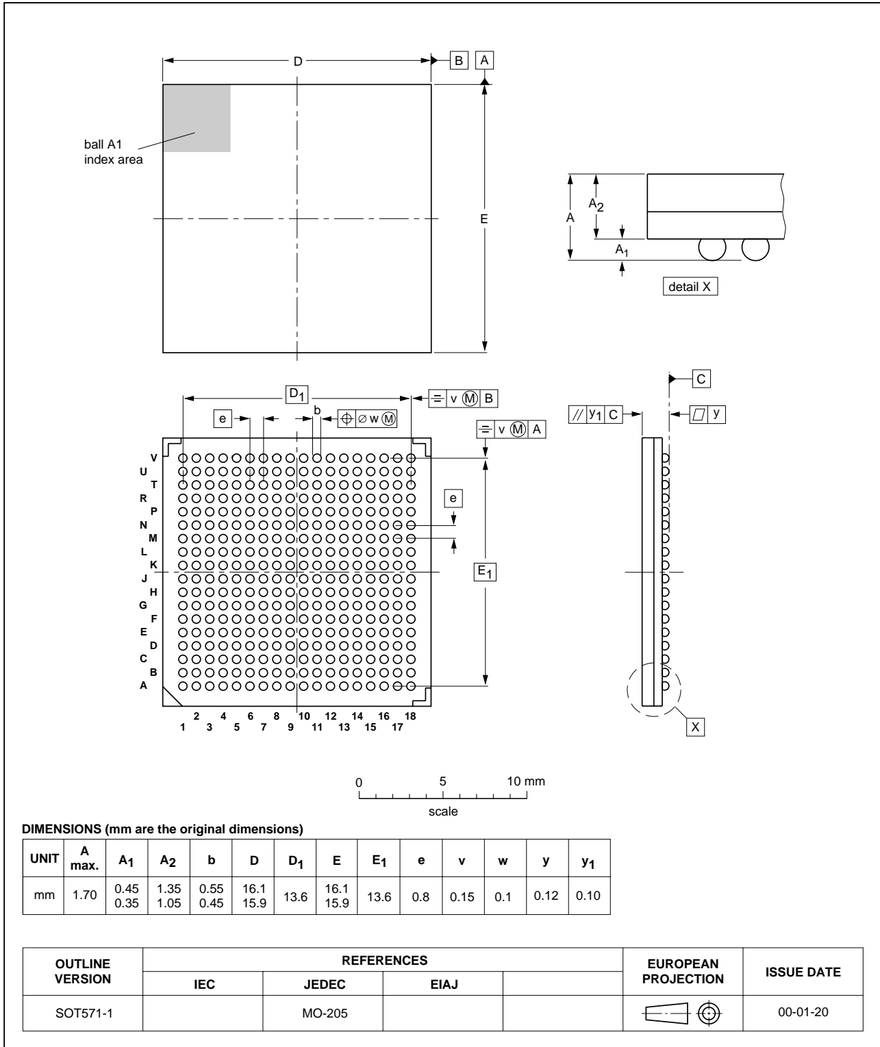
Fig 4. SOT571-1.
